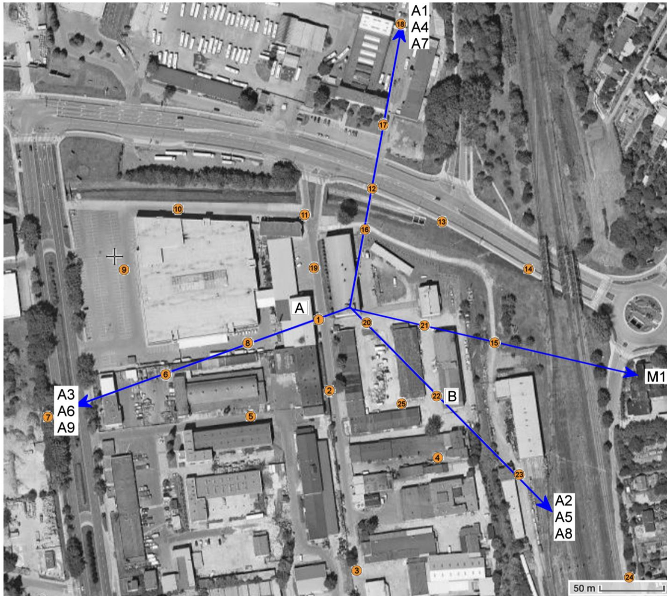
Załącznik nr 2: Lokalizacja anten oraz ich azymuty, lokalizacja pionów (punktów) pomiarowych wokół instalacji radiokomunikacyjnej. Mapa źródłowa: Geoportal. ● -punkt (pion) pomiarowy.
